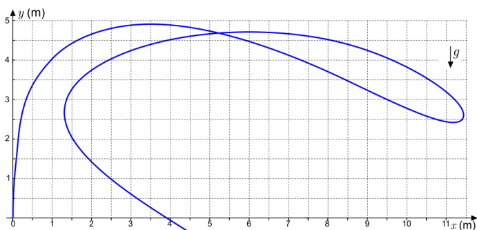
Figur 2: På EuPhO i Riga 2019 såg den tredje teoriuppgiften ut så här: En vattenstråle åker ut ur en vattenslang med en konstant, okänd, fart v . Ett barn leker med slangen genom att låta den rotera i det vertikala xy planet. Utgångshålet hålls fast i läget x = y = 0 m, och vinkeln mellan axeln genom munstycket och horisonten är aldrig mindre än 45^\circ . Strålen har hela tiden en oregelbunden form, och i ett visst ögonblick har den det utseende som visas i figuren. Använd figuren för att bestämma farten v under antagandet att accelerationen vid fritt fall är g = 9,8 \text{ m/s}^2 (figur: EuPhO 23 Academic Committee).
